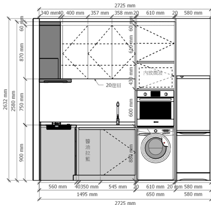
A 立面圖1 02 scale 1:15
